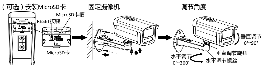
图1-1 壁装
