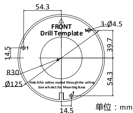
图1-3 安装孔位
