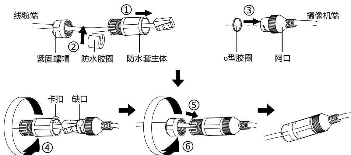
图1-9 安装网口防水套
