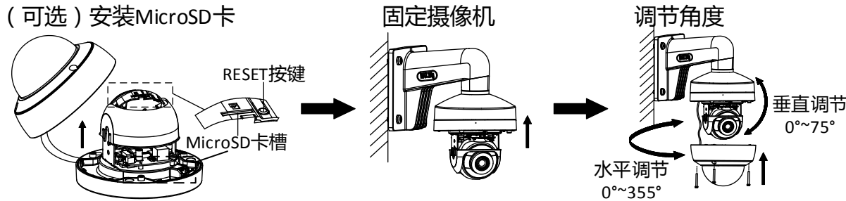
图1-8 壁装
