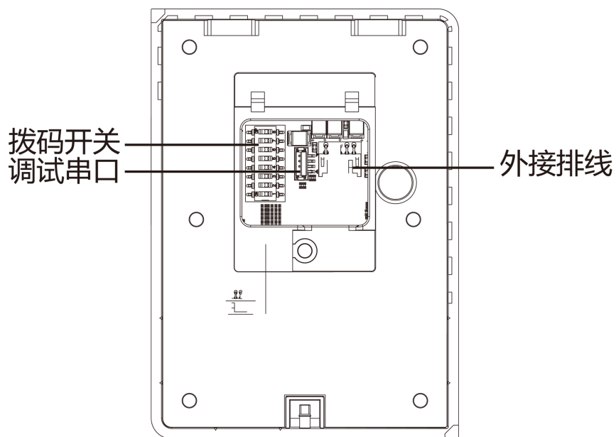
图 2-2 后视图
